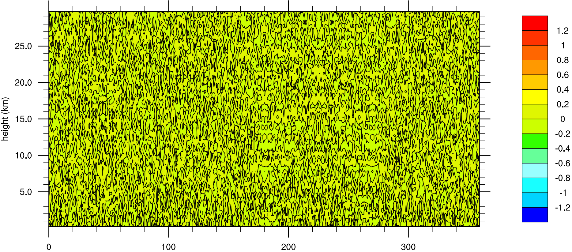
CAM-SE Test 2-1 T' t=0.0 s
