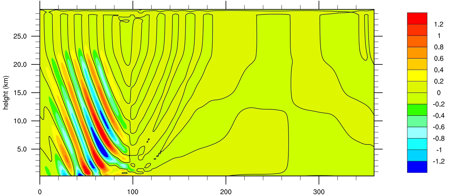
CAM-SE Test 2-1 T' t=7865.0 s
