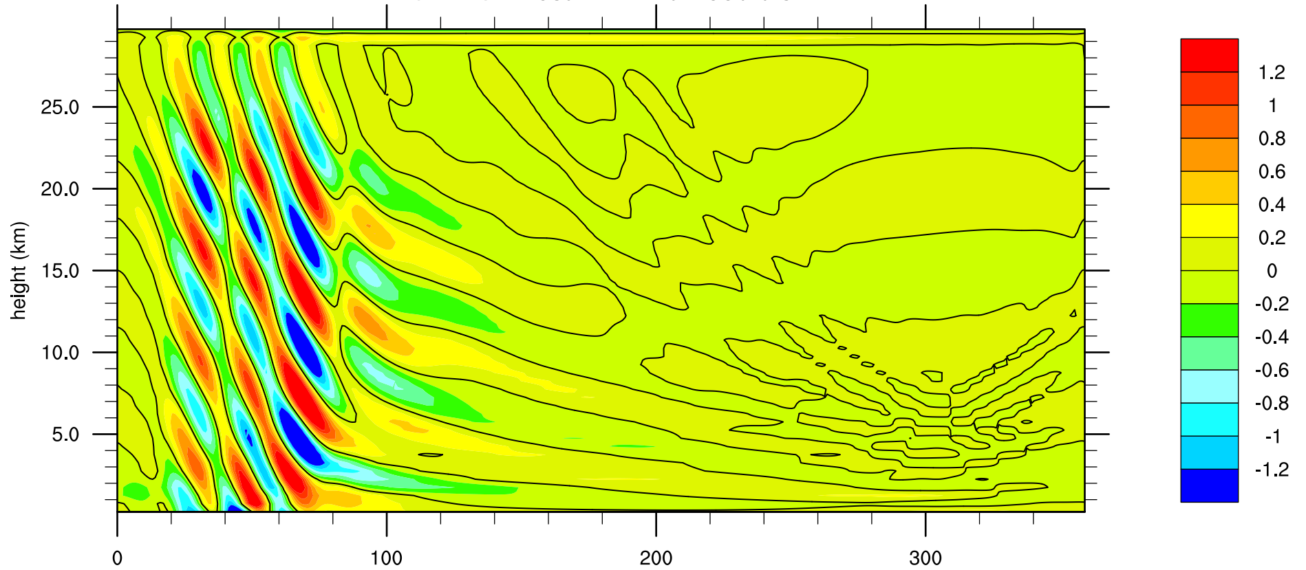
CAM-SE Test 2-1 T' t=2880.0 s
