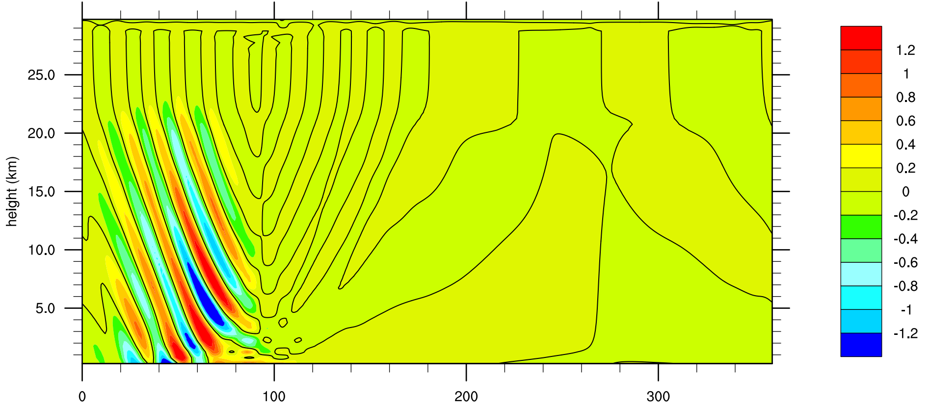
CAM-SE Test 2-1 T' t=7200.0 s
